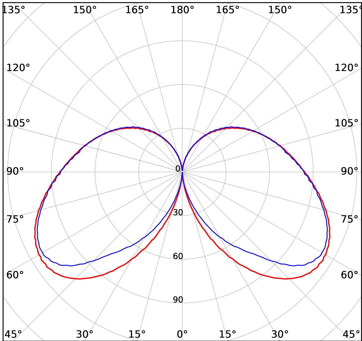
cd 900 lm — C0-C180 — C90-C270
