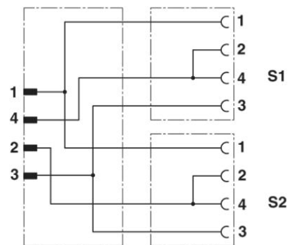
Schaltplan
