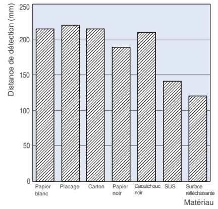
E3ZM-LS□4H(LS□9H)
