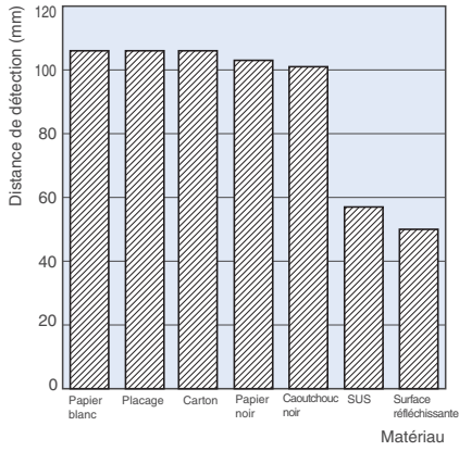
E3ZM-LS□1H(LS□6H)
