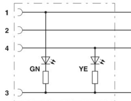
Leitung
