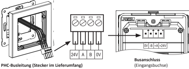
PHC-Busleitung (Stecker im Lieferumfang)
