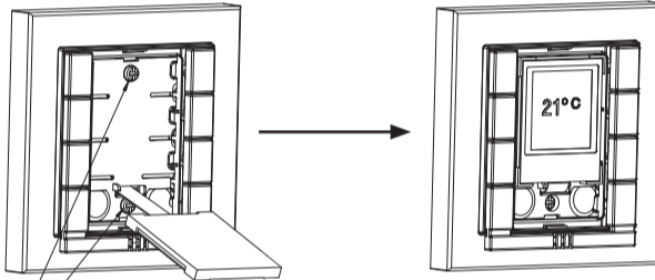
Display vorsichtig herunterklappen und Schrauben leicht festziehen
