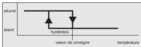
Schéma 2 : régulation à 2 points
