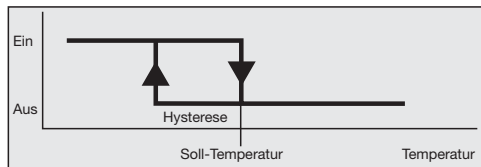
Bild 2: 2-Punkt-Regelung
