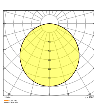
PL CMFT 600 P 30W 865 PS
