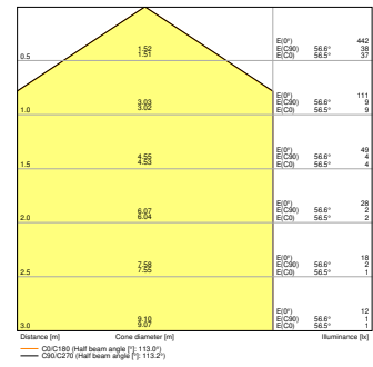
PL CMFT 600 P 33W 865 PS EM CONVERSION BOX
