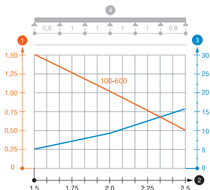
Slodzes diagramma, kabeļu rene, tips MKSMU 60
