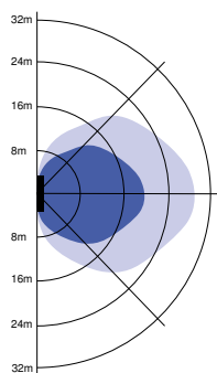
Installatie - Muur montage Aanbevolen installatie hoogte 1-4m
