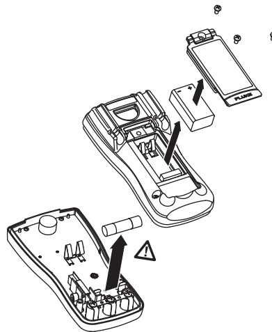
Afbeelding 2. Demontage
