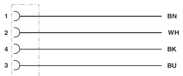
Kontaktbelegung des M12-Steckers und der M12-Buchse
