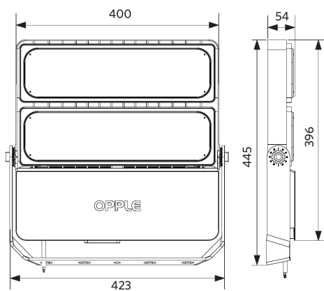
LEDfloodMo-P Re450
